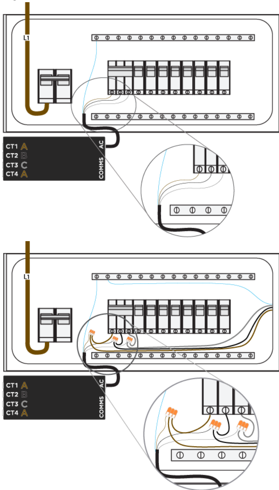
Figura 4. Cavo per la misura dei riferimenti voltmetrici cablato all'interruttore dedicato (superiore) o collegato all'interruttore esistente (inferiore) (trifase)
