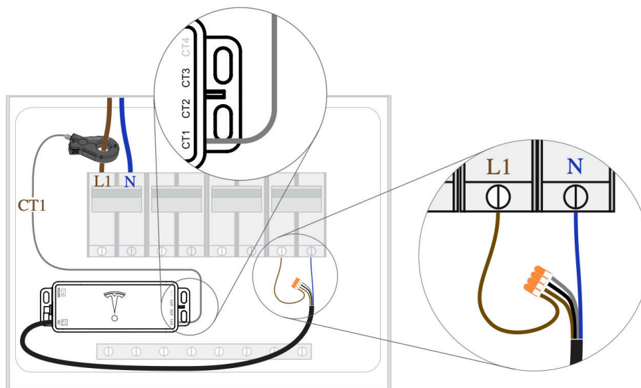
Figura 2. Configurazione del contatore all'interno del pannello - Monofase
