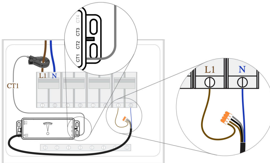
Figur 2. Konfiguration av fjärrmätare inuti panelen – enfas
