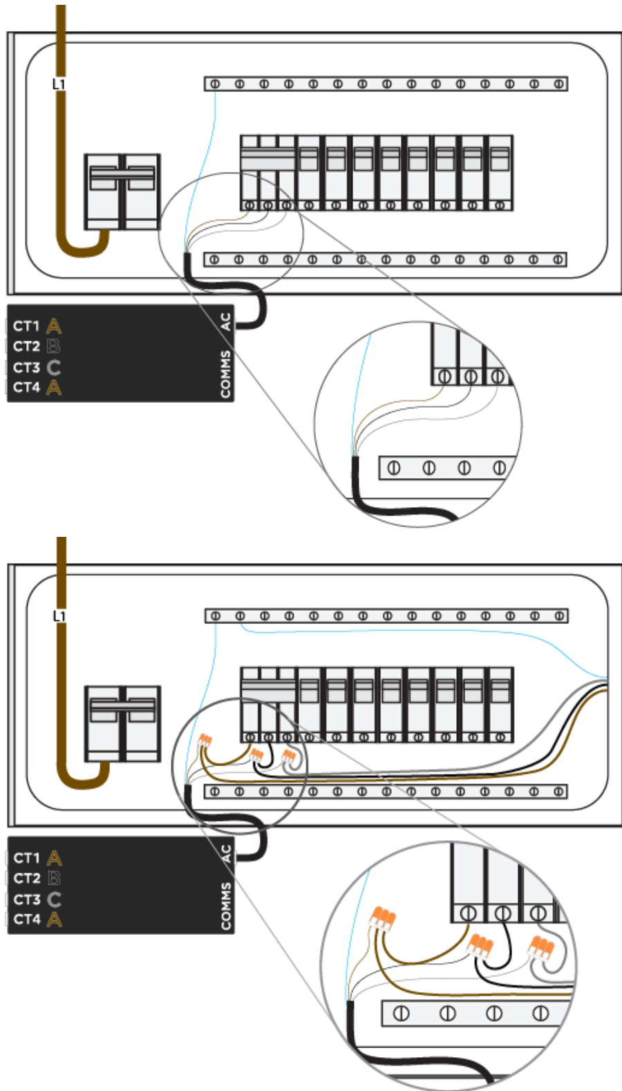
Figur 4. Spänningskablage anslutet till dedikerad brytare (övre) eller skarvat till befintlig brytare (nedre) (trefas)
